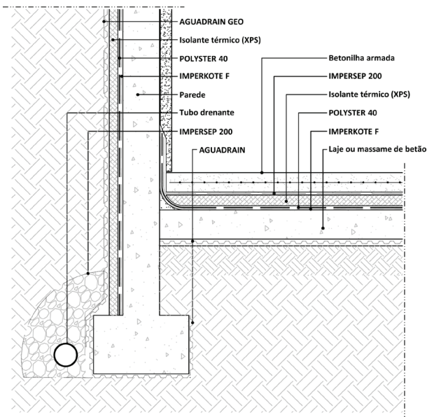
Figura 1 – Aplicação dos revestimentos em paredes e pavimentos em contacto com o terreno
