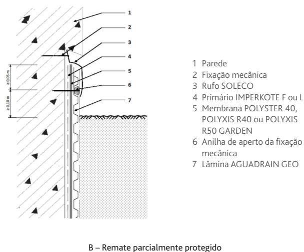
Figura 3 – Remate do bordo superior das membranas numa parede
